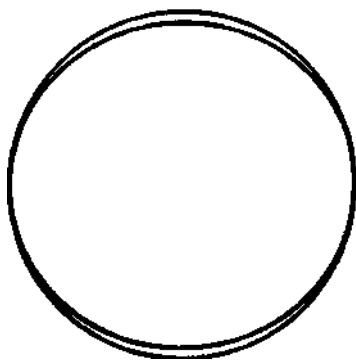
Уплющенность Юпитера
