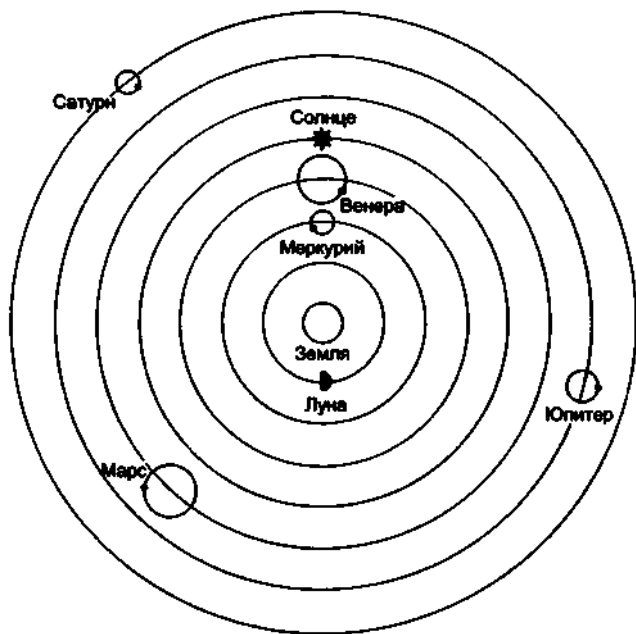
Система Птолемея
